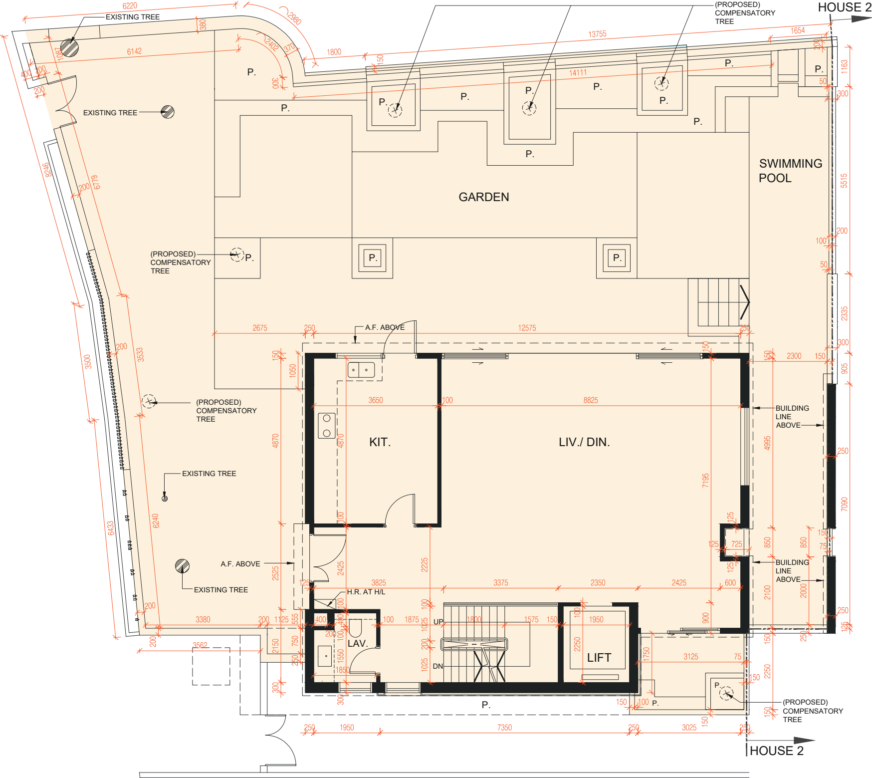
GROUND FLOOR PLAN 地下平面圖
